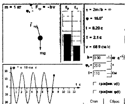
Рис. 5.4. Модель математического маятника
